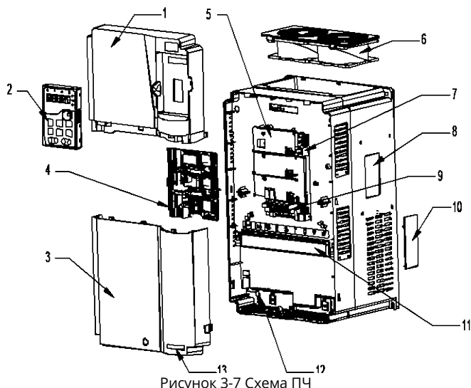
Рисунок 3-7 Схема ПЧ
