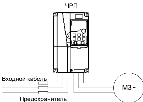
Рисунок 4-24 Конфигурация предохранителя
