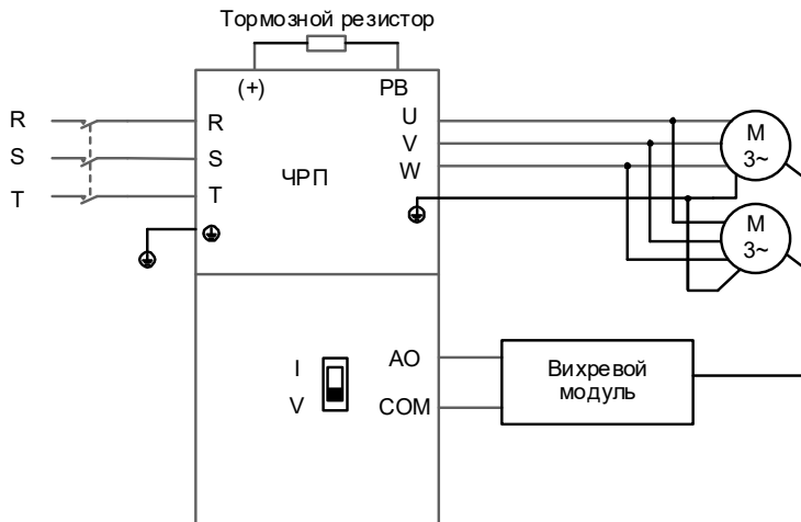
Рисунок 5-6 Подключение клеммы АО к вихревому модулю
