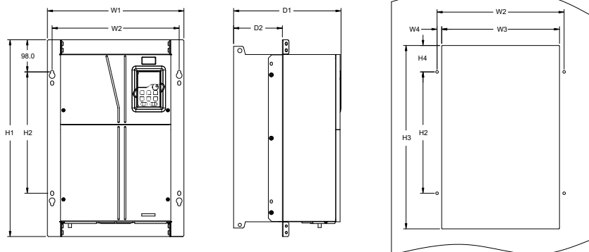
Рисунок С-20 Схема фланцевого монтажа ПЧ 660 В мощностью 22–132 кВт
