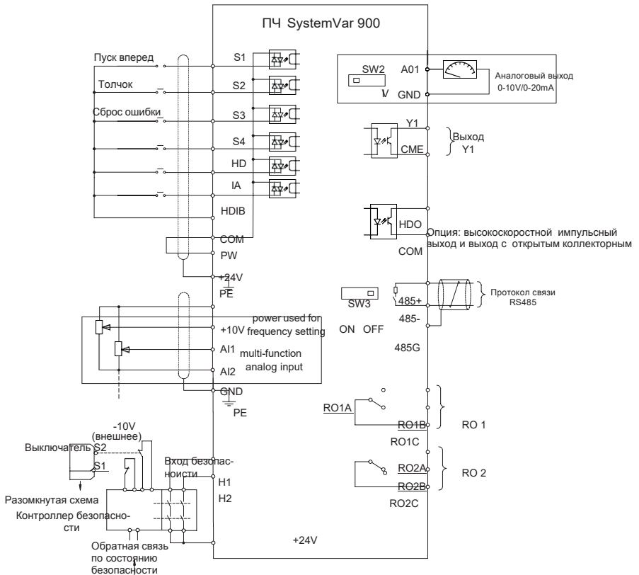
Рис 4.17 Схема подключения цепей управления
