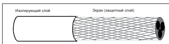
Сечение кабеля
