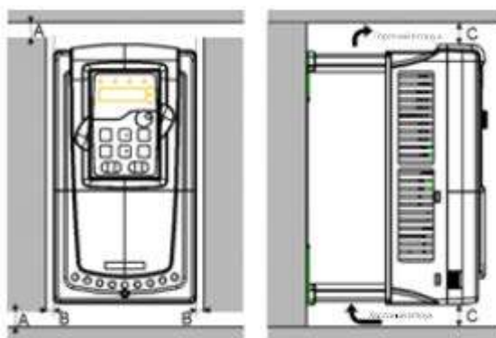
Рис. 4-2 Место установки
