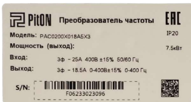
Рисунок 2-1. Шильдик преобразователей частоты PAC0200
