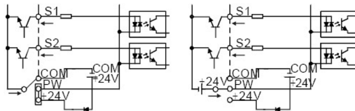
Рис.5-19 NPN режим
