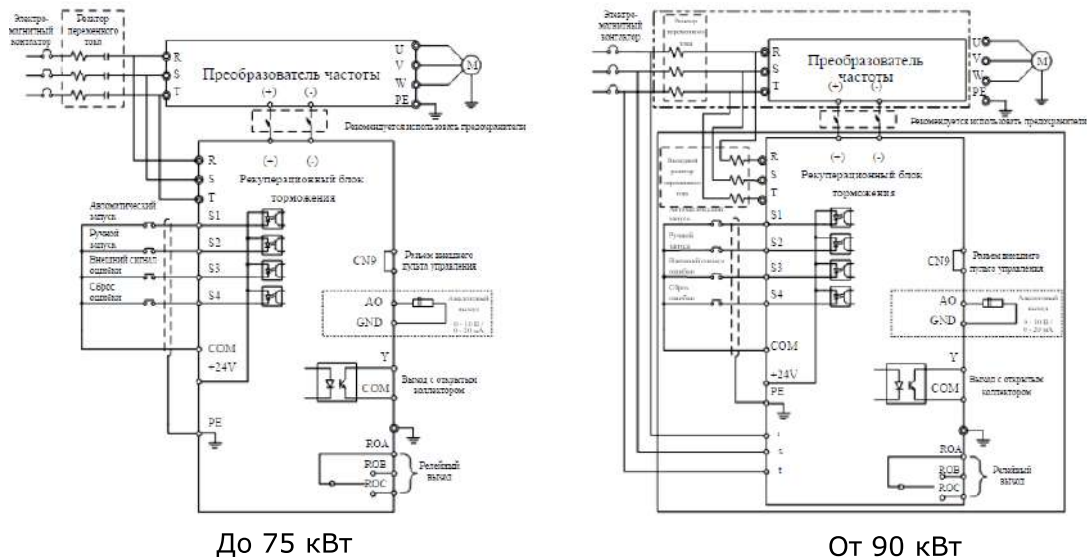
Рис. 12-4. Схема подключения модуля PEOPRBU
