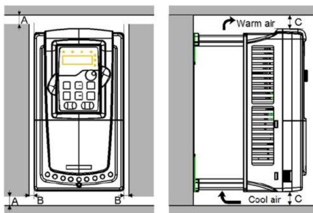
Рисунок 4-16. Вентиляционные промежутки
