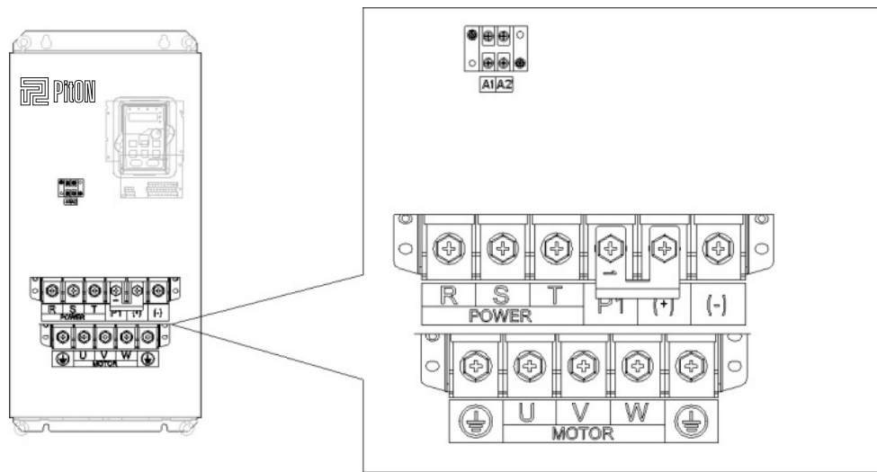
Рис. 5-10 Клеммы силовых цепей 75 – 110 кВт
