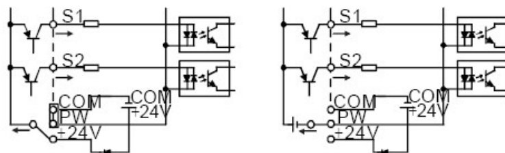
Рис.5-20 PNP режим
