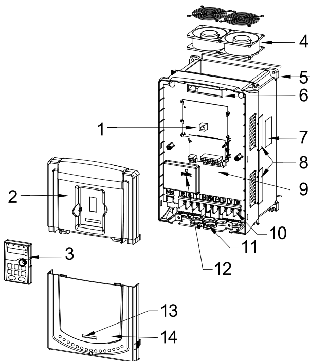
Рисунок 3-1. Структурная схема преобразователя частоты PAC0200.
