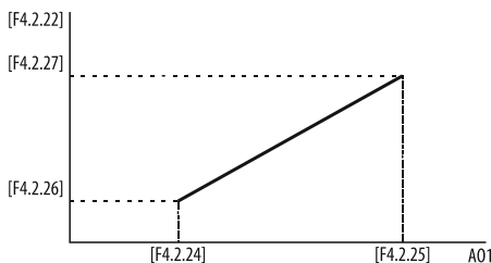
Рисунок 117 – масштабирование значения параметра мониторинга относительно диапазона выходного сигнала на выходе А01.
