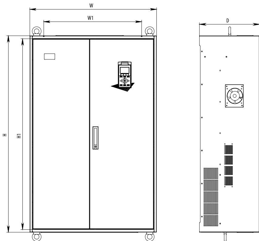
Рисунок 16 - габаритные размеры AFD-E2500.43 и выше (тип корпуса 4, габарит 13)
