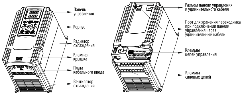
Рисунок 4 – тип корпуса 2, габариты 3, 4, 5, 6, 7 (модели AFD-E055.43В...AFD-E300.43)
