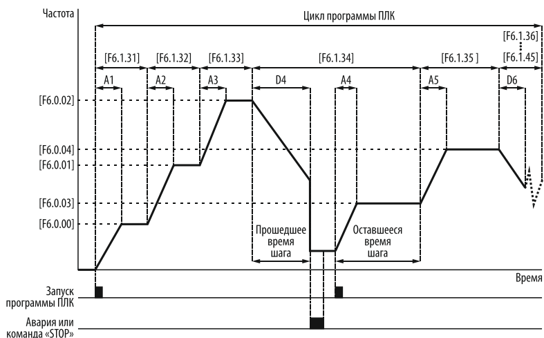
Рисунок 157 – запуск программы ПЛК с частоты шага прерывания программы.
