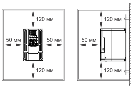
Рисунок 9 – минимально допустимые расстояния от ПЧ до окружающих предметов.
