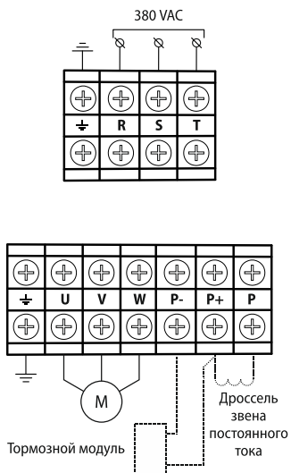
Рисунок 32 - клеммы силового терминала (модификации: AFD-E2500.43, AFD-E2800.43, AFD-E3150.43)
