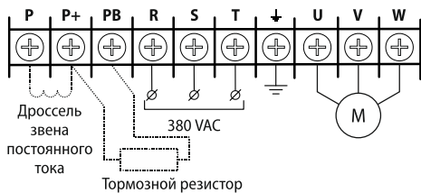
Рисунок 27 - клеммы силового терминала (модификации: AFD-E220.43B)
