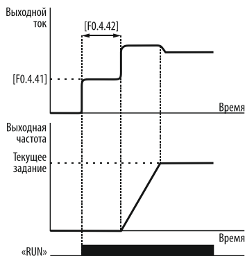
Рисунок 79 – запуск электродвигателя с предвозбуждением.
