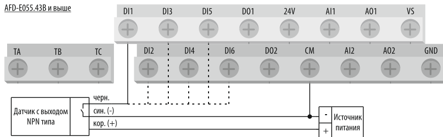
Рисунок 39 – схема подключения датчиков с выходом NPN типа к дискретным входам (питание от внешнего источника питания 24 В).
