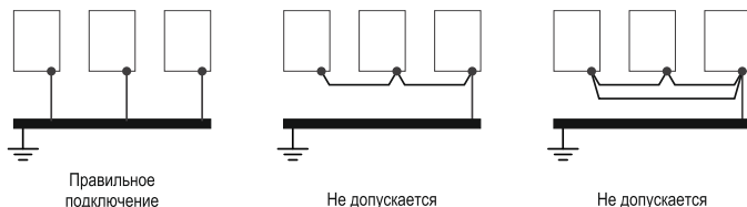
Рисунок 20 – рекомендуемая схема заземления нескольких ПЧ
