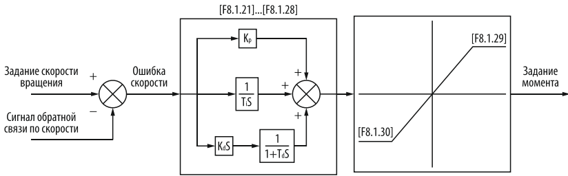
Рисунок 166 – блок-схема регулятора скорости.
