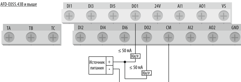
Рисунок 48 – схема подключения нагрузки к транзисторному выходу (питание от внешнего источника питания 24 В).
