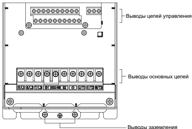
Рис. 3-14. Конфигурация выводов
