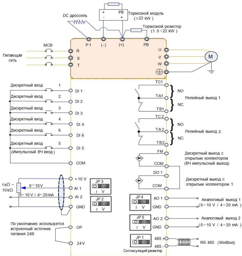
Рис.3.4- Принципиальная электрическая схема подключения.
