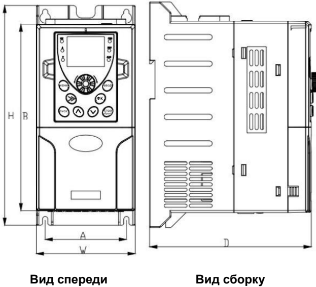
Рисунок 2-1. Габаритные и монтажные размеры преобразователя частоты.
