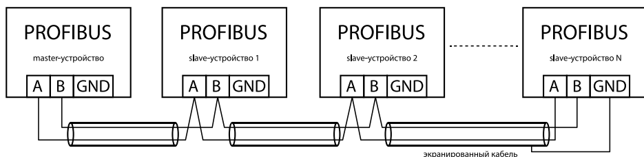
Рисунок 2 – Схема подключения сети Profibus
