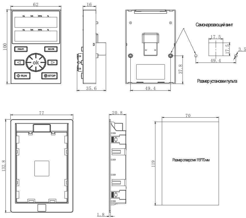
AC310 Форма внешнего кармана клавиатуры и размер отверстия
