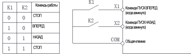
0: Двухпроводное управление 1 схема
