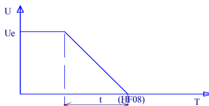
Рис.5 Плавная остановка
