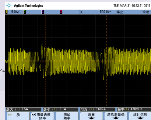
Форма тока в режиме векторного управления без обратной связи с полной нагрузкой на частоте 50 Гц.
