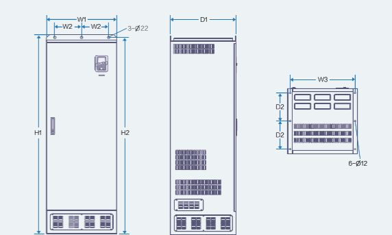
Напольный монтаж преобразователей 350—500кВт
