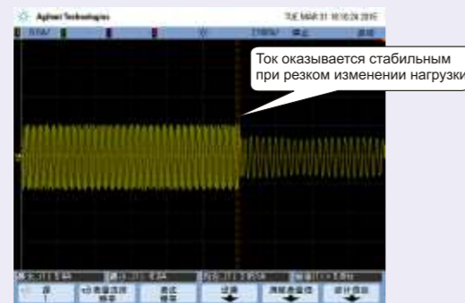
Форма тока при внезапной разгрузке в режиме скалярного управления с полной нагрузкой на частоте 2 Гц.
