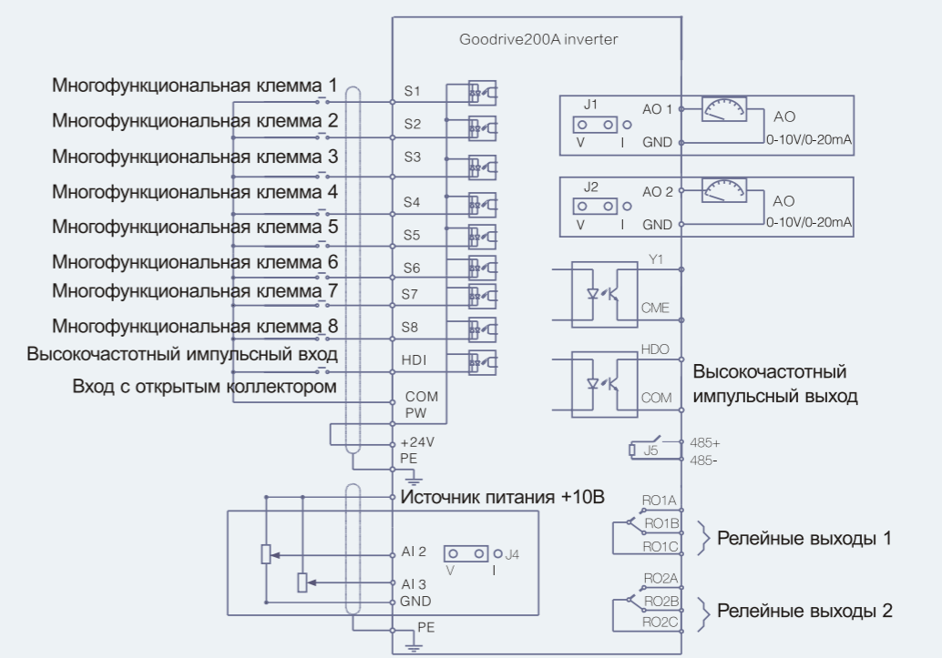
Схема подключения цепи управления
